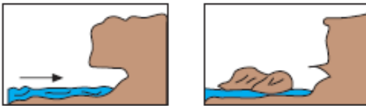
Falezin oluşumu
