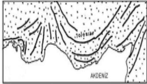
Boyuna kıyılar
