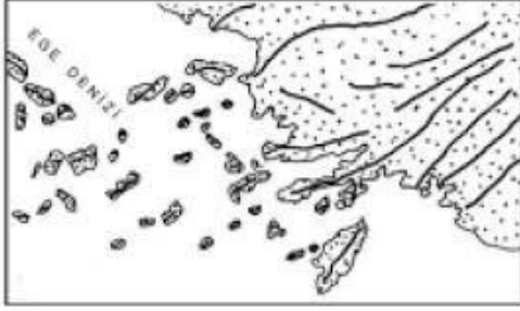
Enine kıyılar
